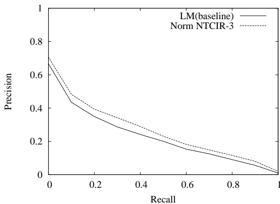
図 2: 再現率精度グラフ (NTCIR-3)
