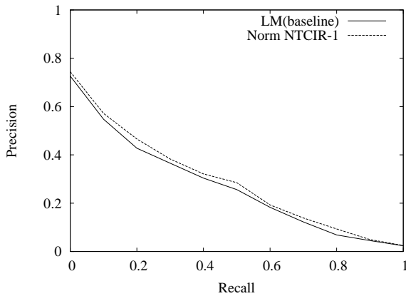
図 1: 再現率精度グラフ (NTCIR-1)
