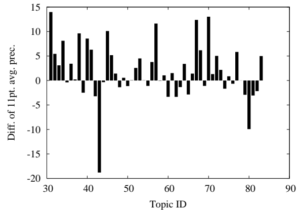
図 3: 検索課題ごとの性能差 (NTCIR-1)
